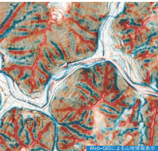
Web-GISによる山地情報表示
