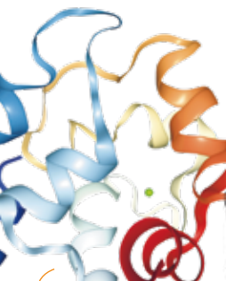
タンパク質の立体構造
